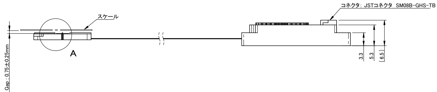
詳細図 A スケール 5 : 1
