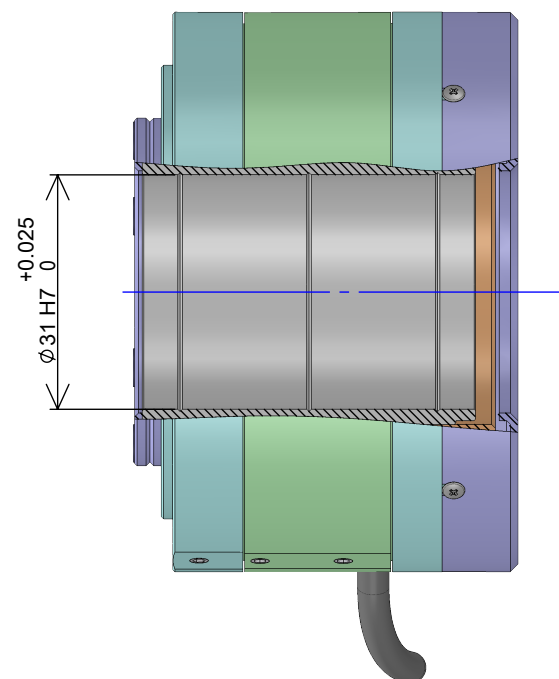
ロータ断面図
